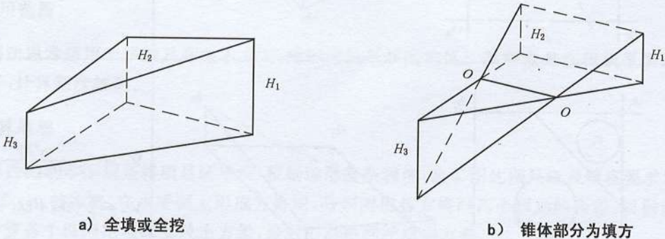
图 B.2 三角棱柱体的体积计算
